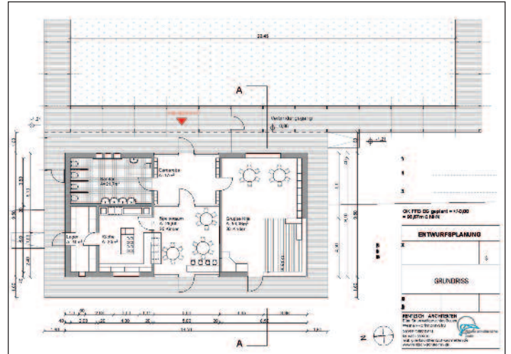
Grundriss Erweiterungsbau
